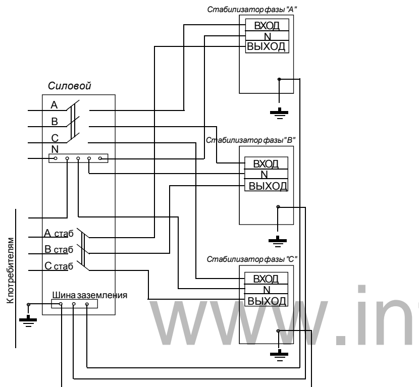
Рисунок 4 - Схема подключения стабилизатора в трехфазной сети
