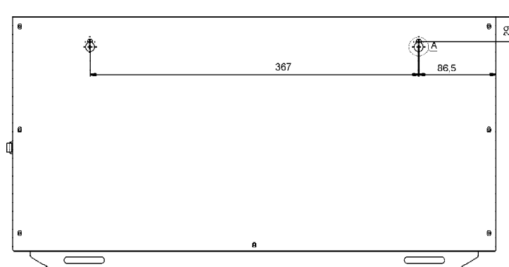
Габаритные и установочные размеры стабилизатора напряжения переменного тока LIDER PS12000W-50
