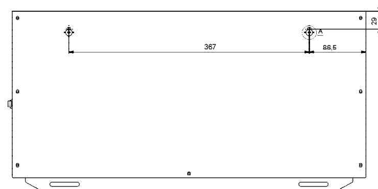
Габаритные и установочные размеры стабилизатора напряжения переменного тока LIDER PS3000SQ-C-15
