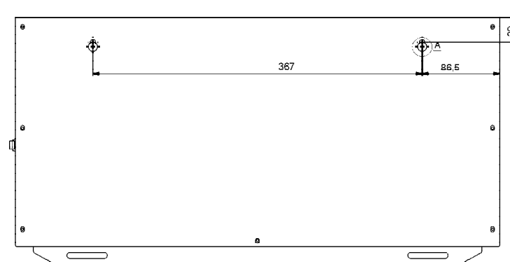
Габаритные и установочные размеры стабилизатора напряжения переменного тока LIDER PS3000SQ-C-25
