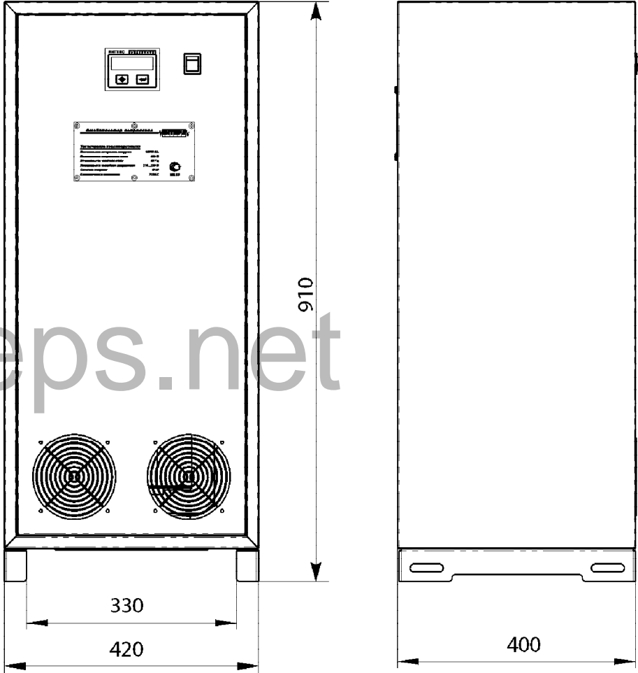
Габаритные и установочные размеры стабилизатора напряжения переменного тока LIDER PS5000SQ-C-40 .
