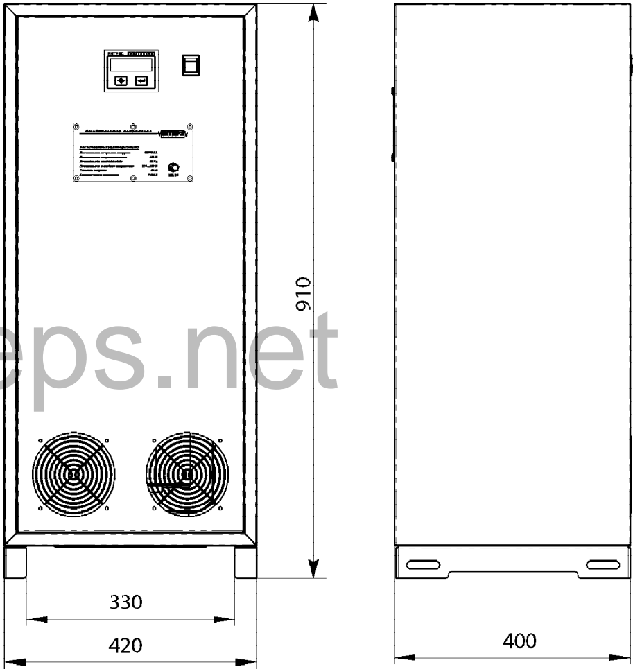
Габаритные и установочные размеры стабилизатора напряжения переменного тока LIDER PS7500SQ-C-25 .
