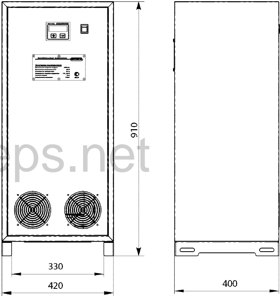
Габаритные и установочные размеры стабилизатора напряжения переменного тока LIDER PS7500SQ-C-40 .
