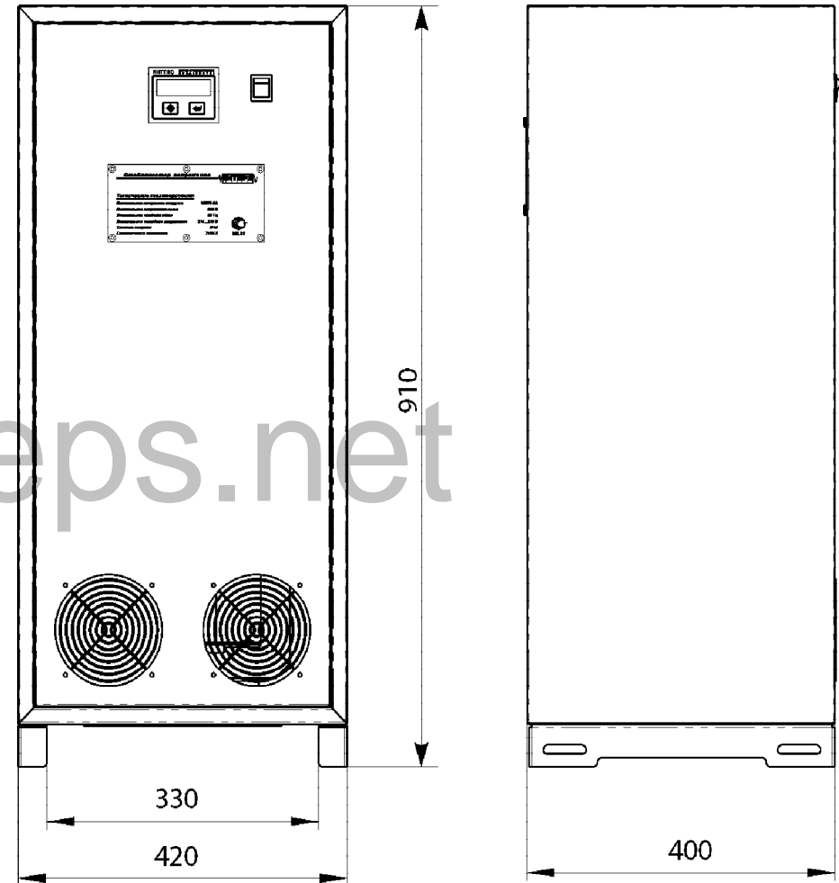
Габаритные и установочные размеры стабилизаторов напряжения переменного тока LIDER PS10000SQ-I-40
