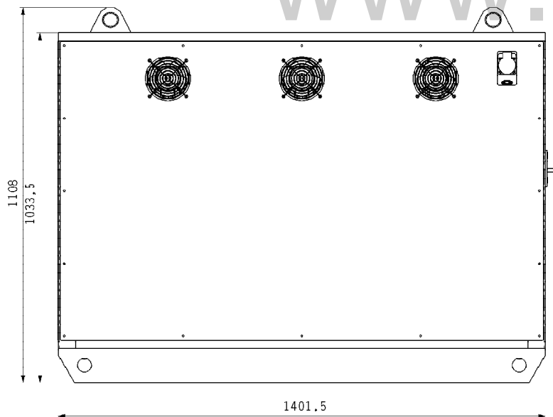
Габаритные и установочные размеры стабилизаторов напряжения переменного тока LIDER PS160000SQ-IM-15
