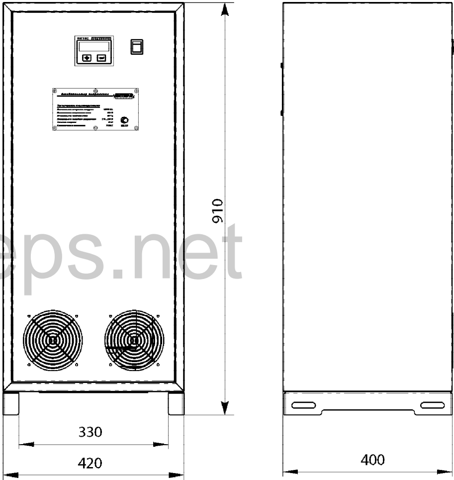
Габаритные и установочные размеры стабилизатора напряжения переменного тока LIDER PS5000SQ-C-25 .
